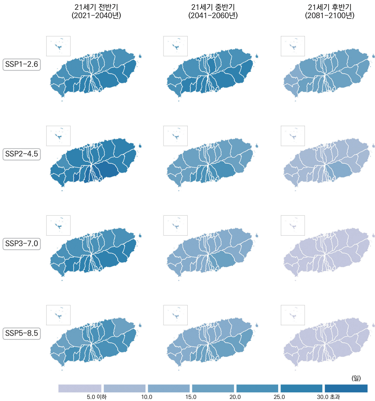
그림 4-30. 제주특별자치도의 한랭일(일) 전망 분포도
