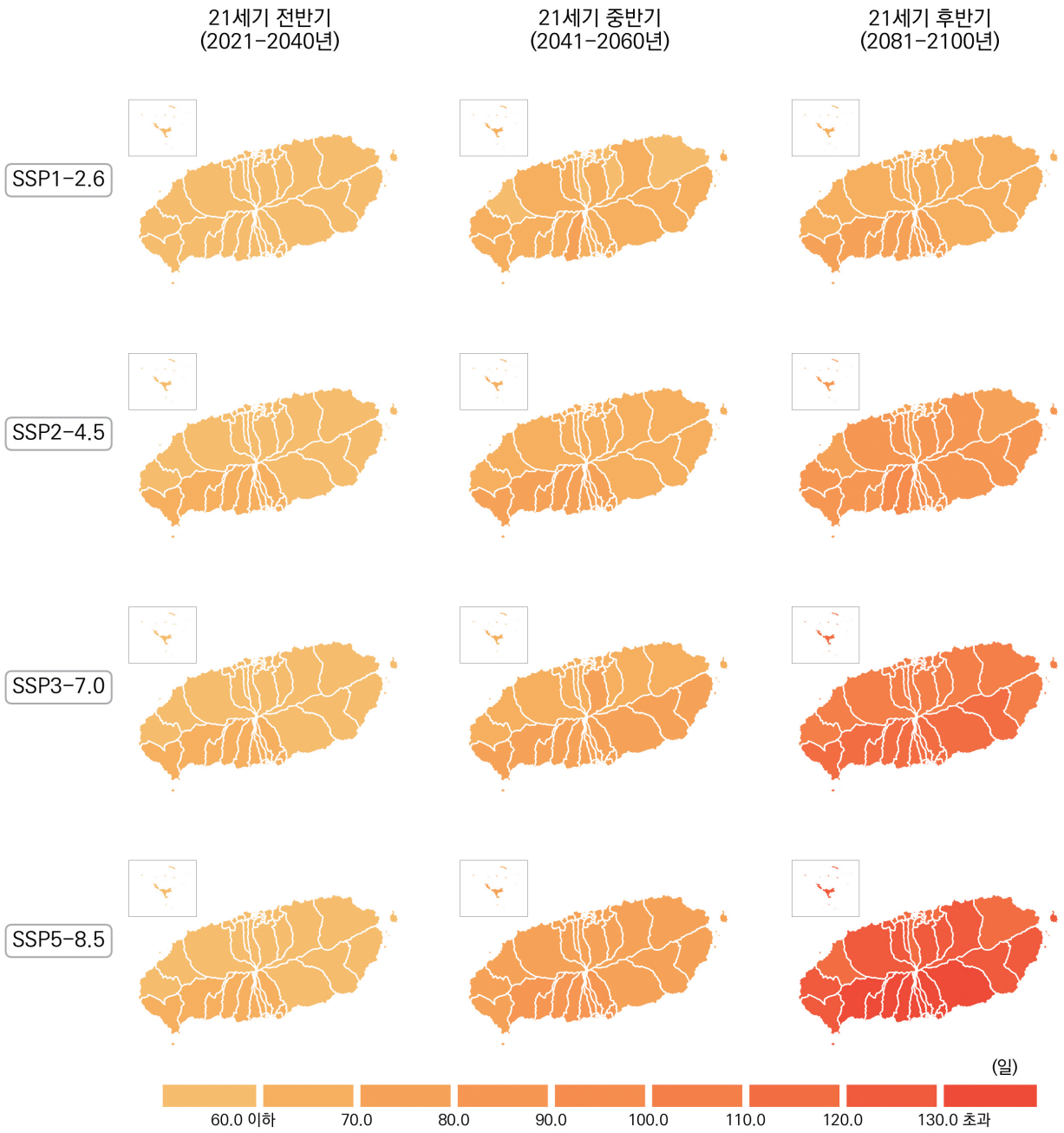
그림 4-21. 제주특별자치도의 온난일(일) 전망 분포도
