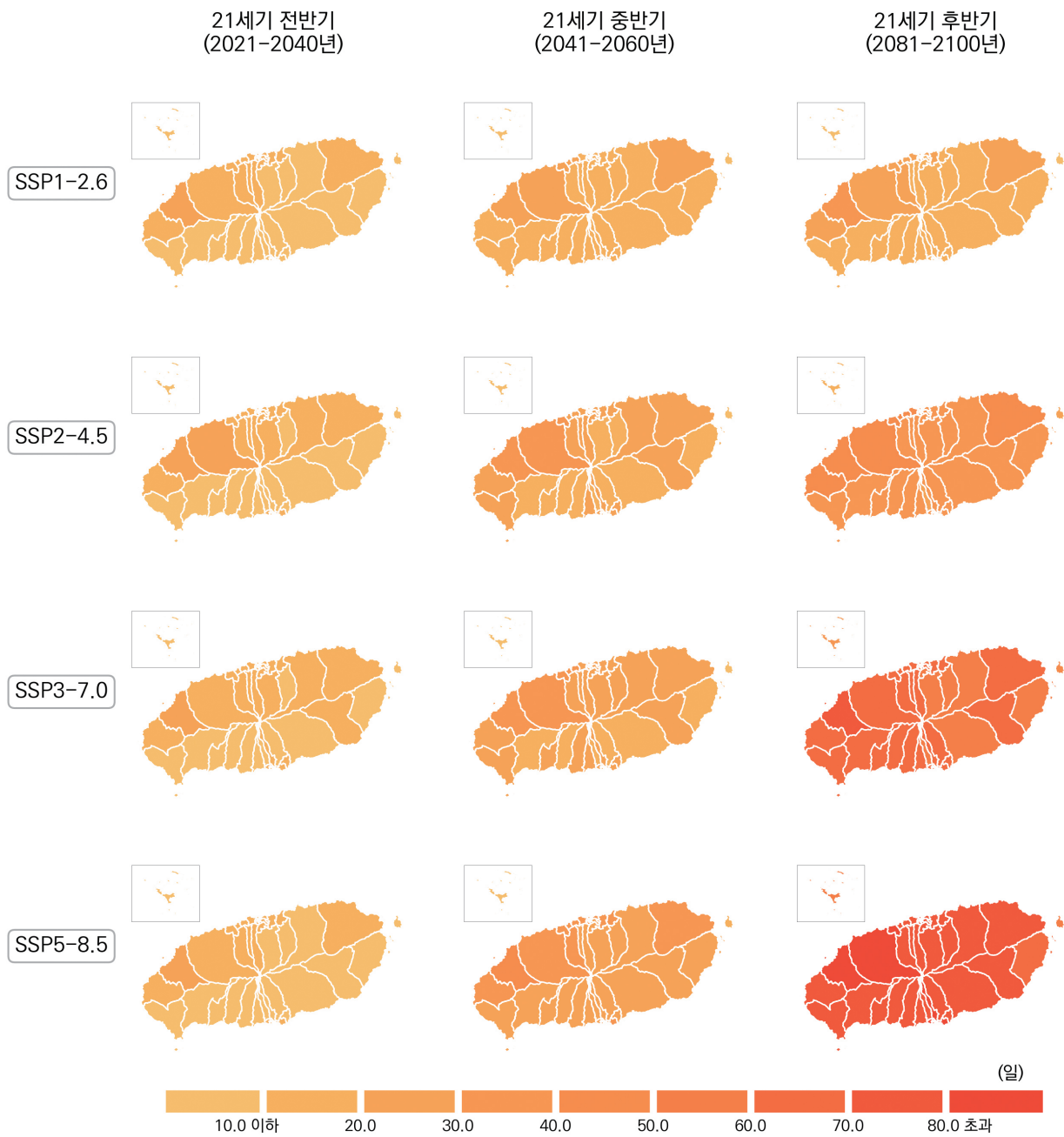
그림 4-18. 제주특별자치도의 폭염일수(일) 전망 분포도
