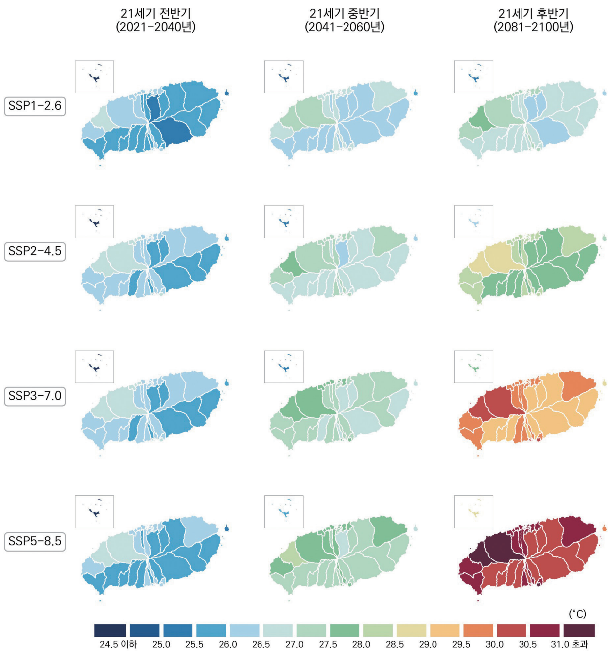
그림 4-3. 제주특별자치도의 여름철 연평균기온(°C) 전망 분포도
