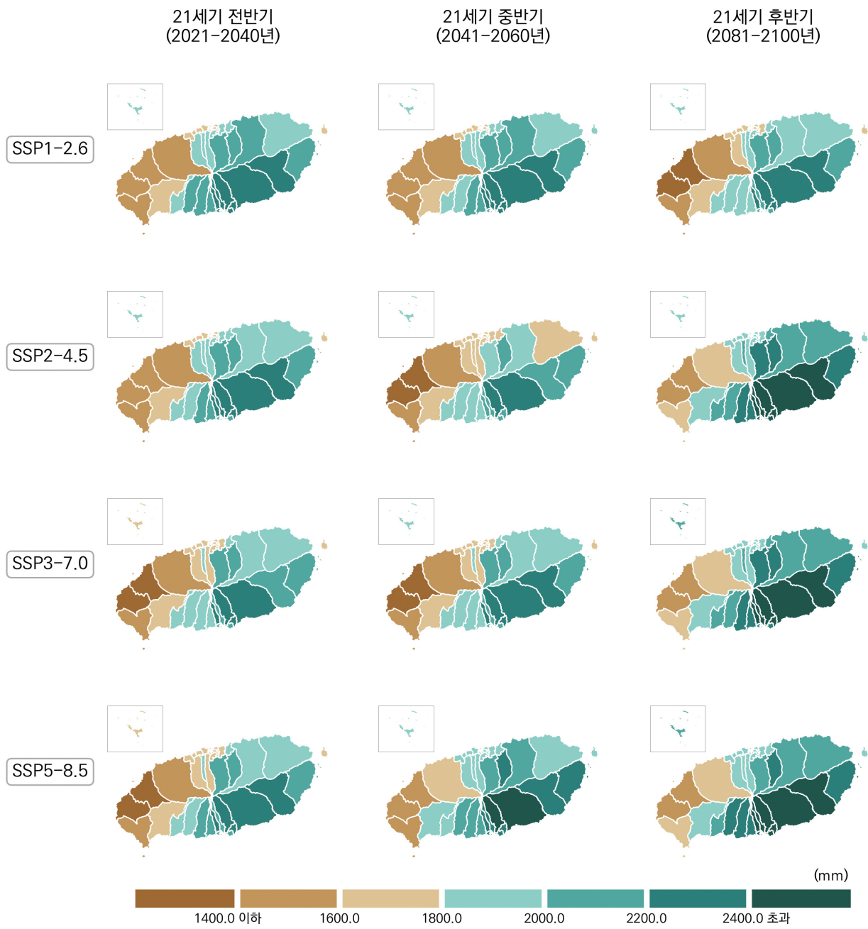
그림 4-16. 제주특별자치도의 연강수량(mm) 전망 분포도
