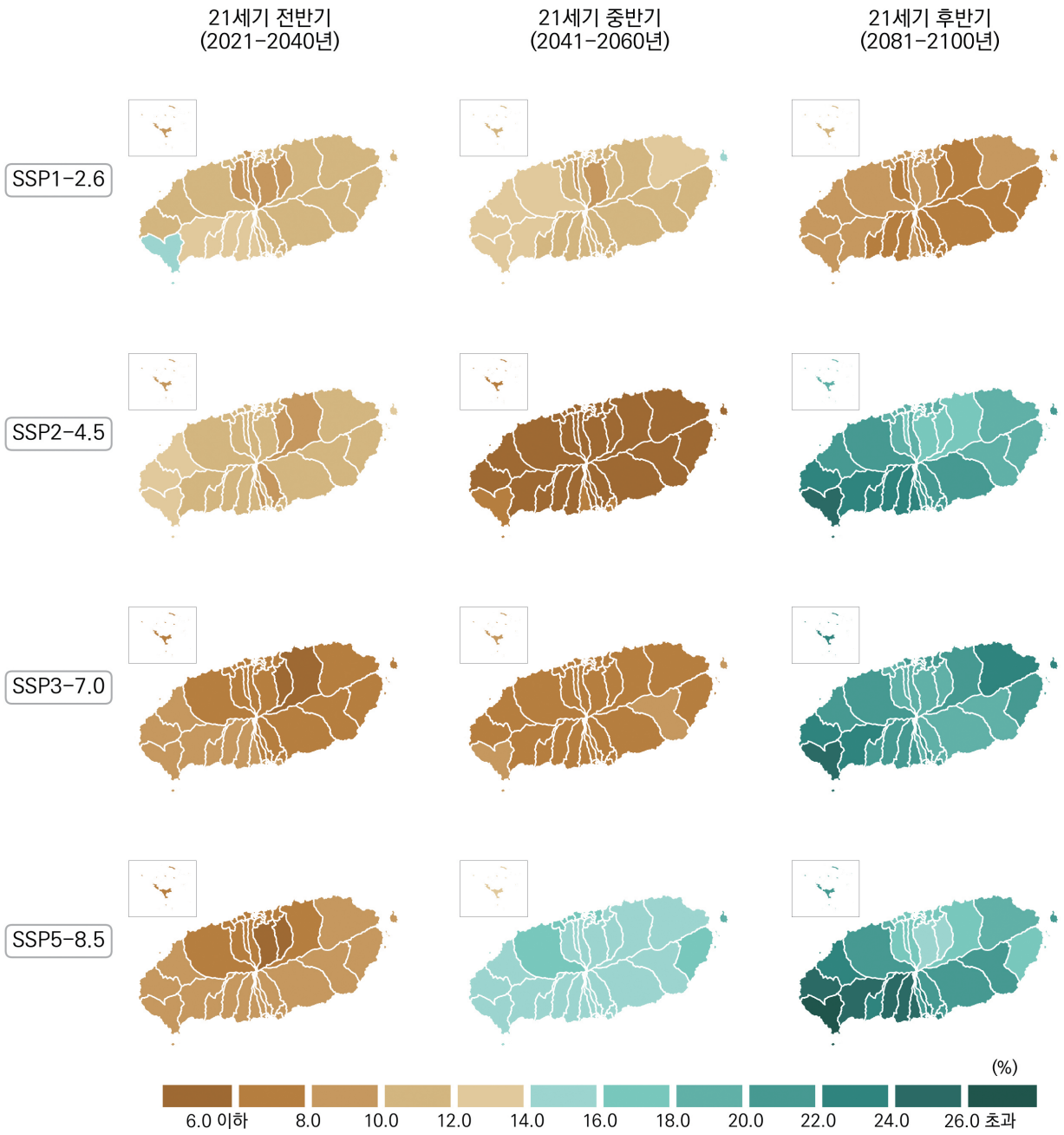
그림 4-17. 제주특별자치도의 연강수량 변화율(%)(2000-2019년 대비) 전망 분포도
