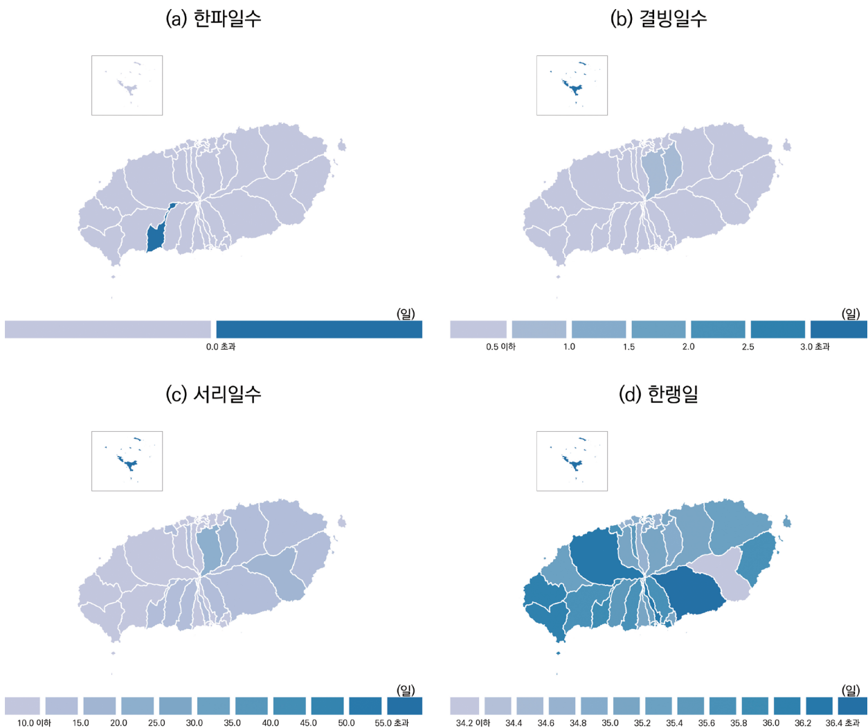
그림 3-3. 현재(2000-2019년) 제주특별자치도 저온 관련 극한기후지수 분포
