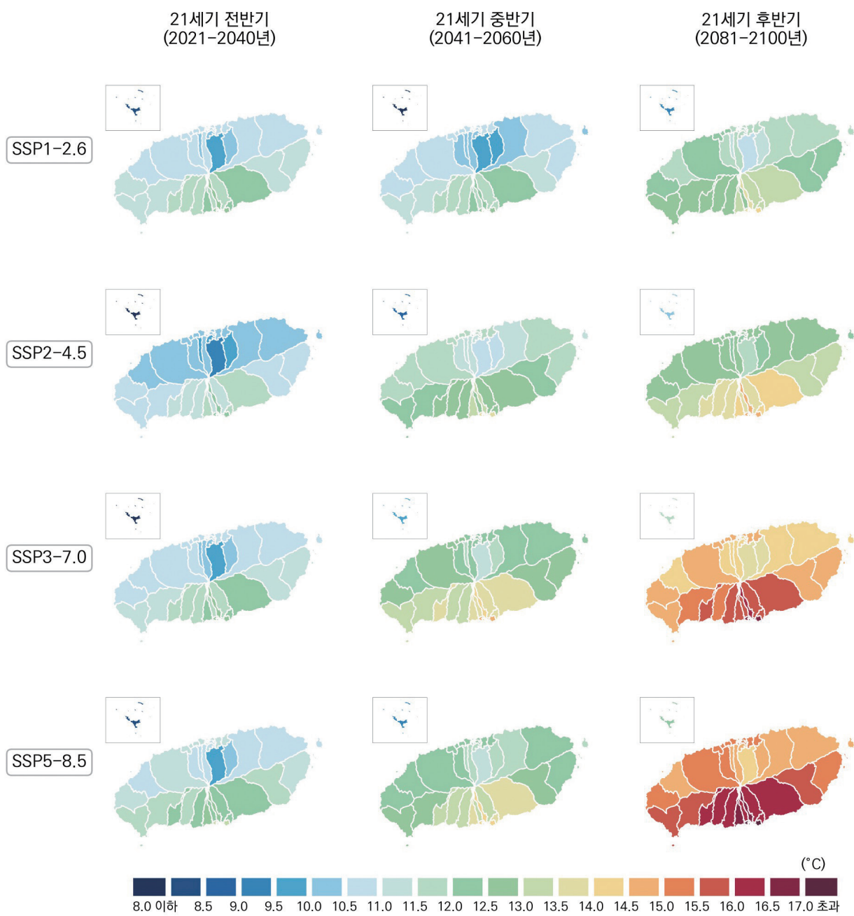
그림 4-10. 제주특별자치도의 겨울철 연평균 최고기온(°C) 전망 분포도
