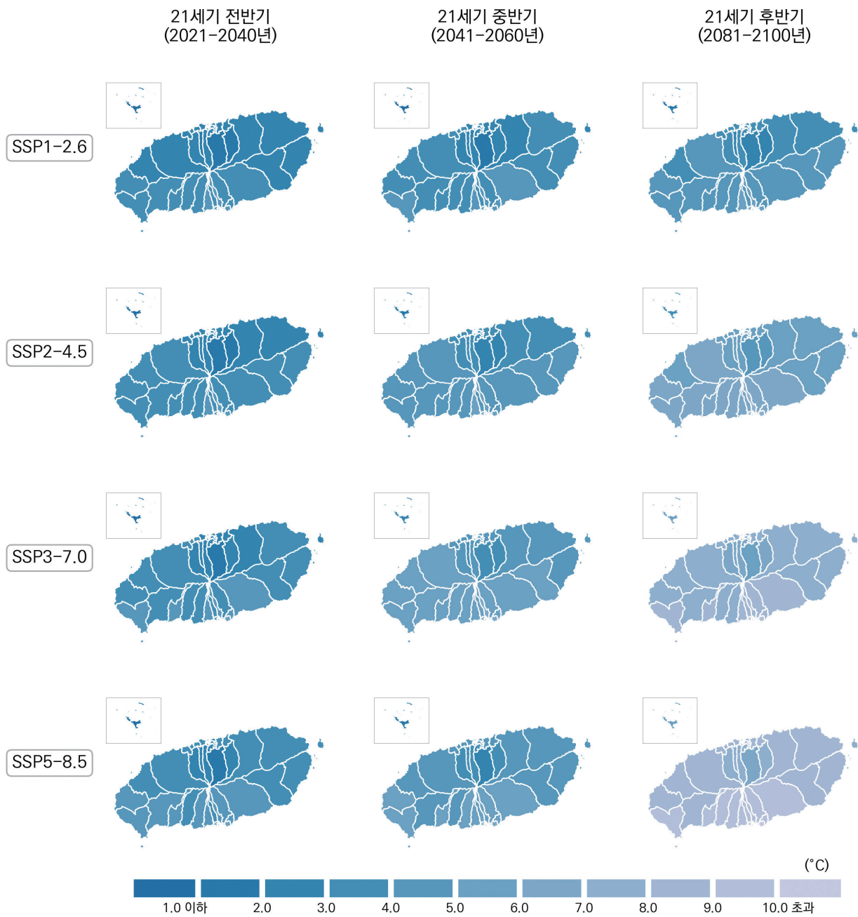
그림 4-32. 제주특별자치도의 일최고기온 연최소(°C) 전망 분포도
