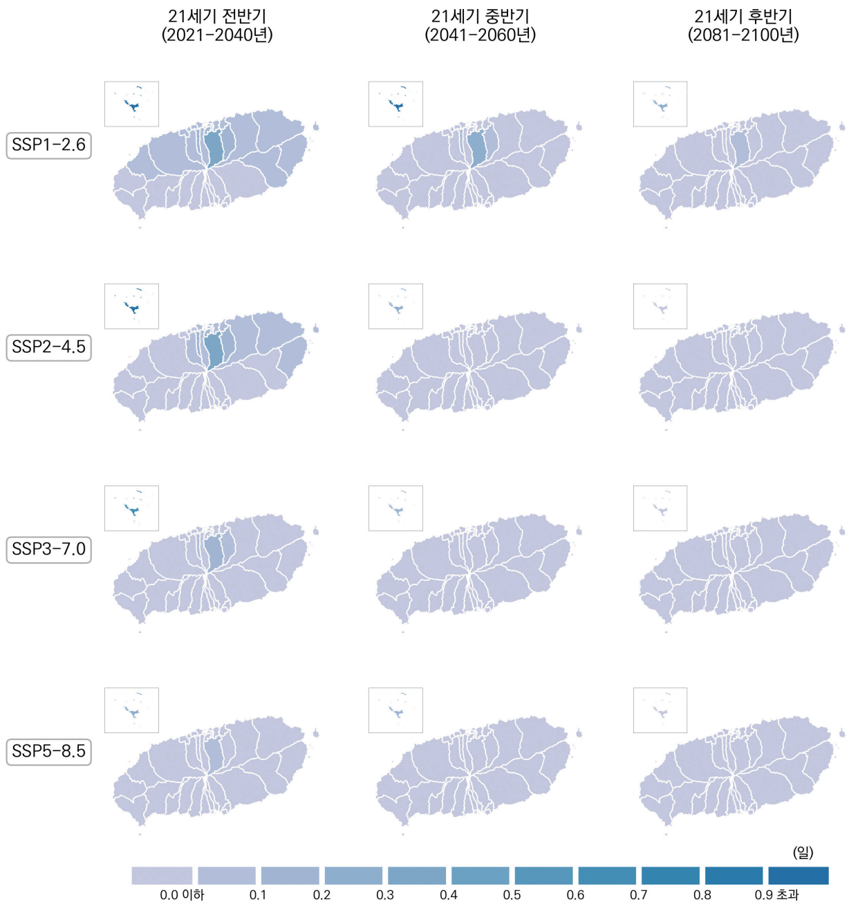
그림 4-28. 제주특별자치도의 결빙일수(일) 전망 분포도
