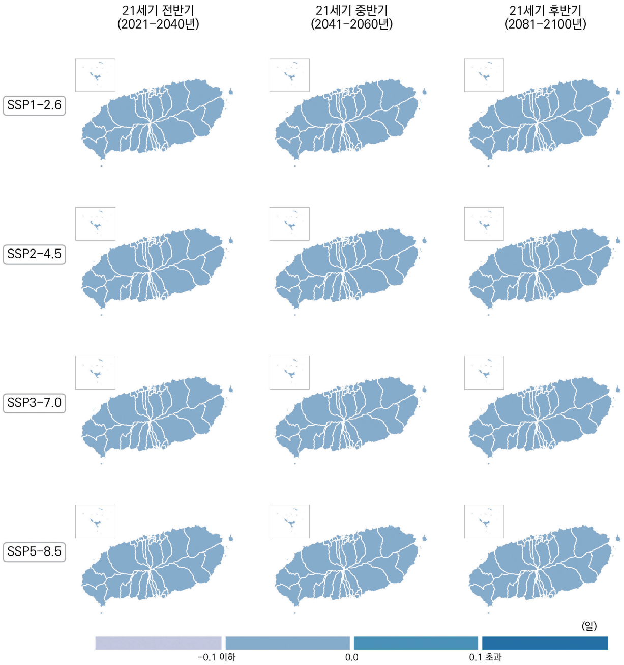
그림 4-27. 제주특별자치도의 한파일수(일) 전망 분포도
