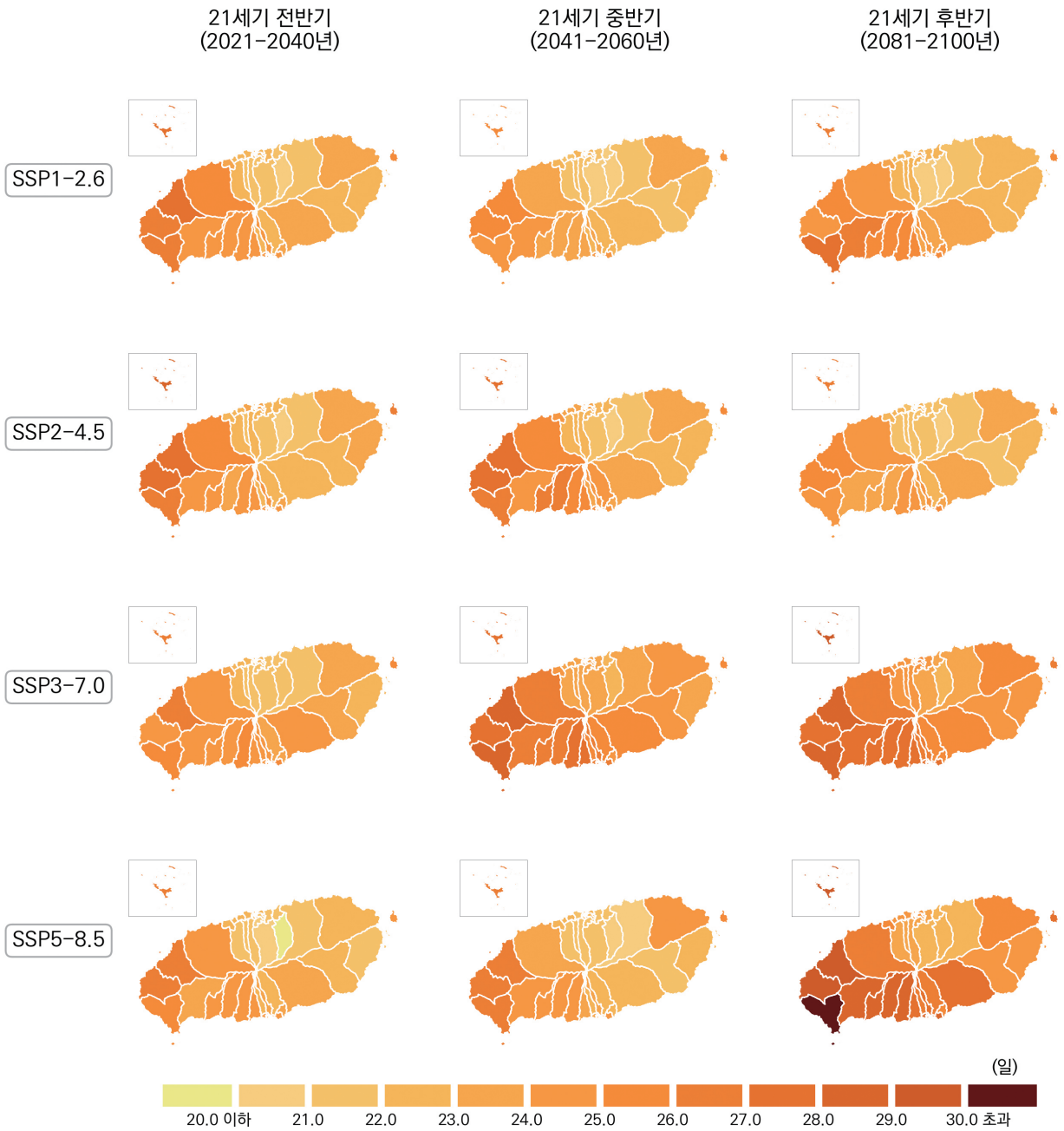
그림 4-40. 제주특별자치도의 최대무강수지속기간(일) 전망 분포도
