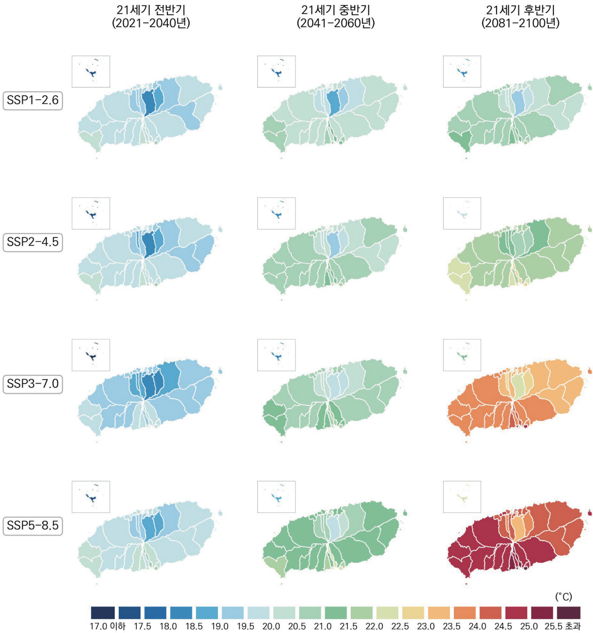
그림 4-4. 제주특별자치도의 가을철 연평균기온(°C) 전망 분포도
