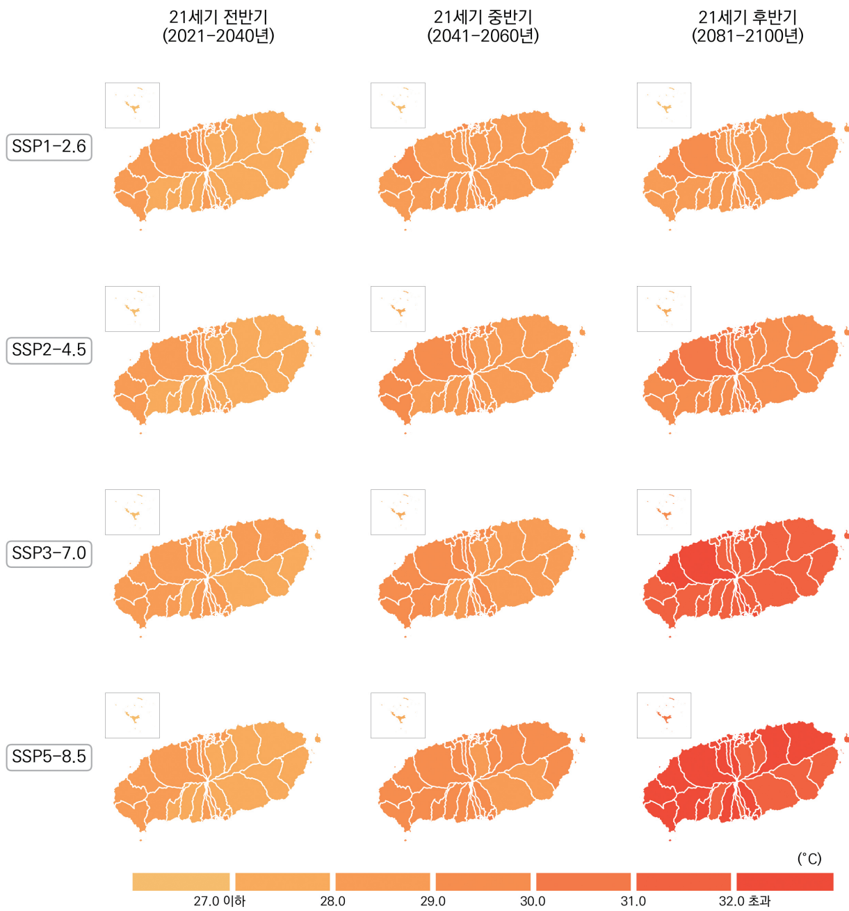
그림 4-24. 제주특별자치도의 일최저기온 연최대(°C) 전망 분포도
