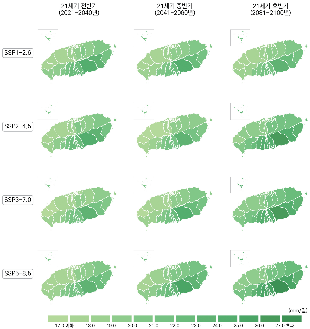
그림 4-35. 제주특별자치도의 강수강도(mm/일) 전망 분포도
