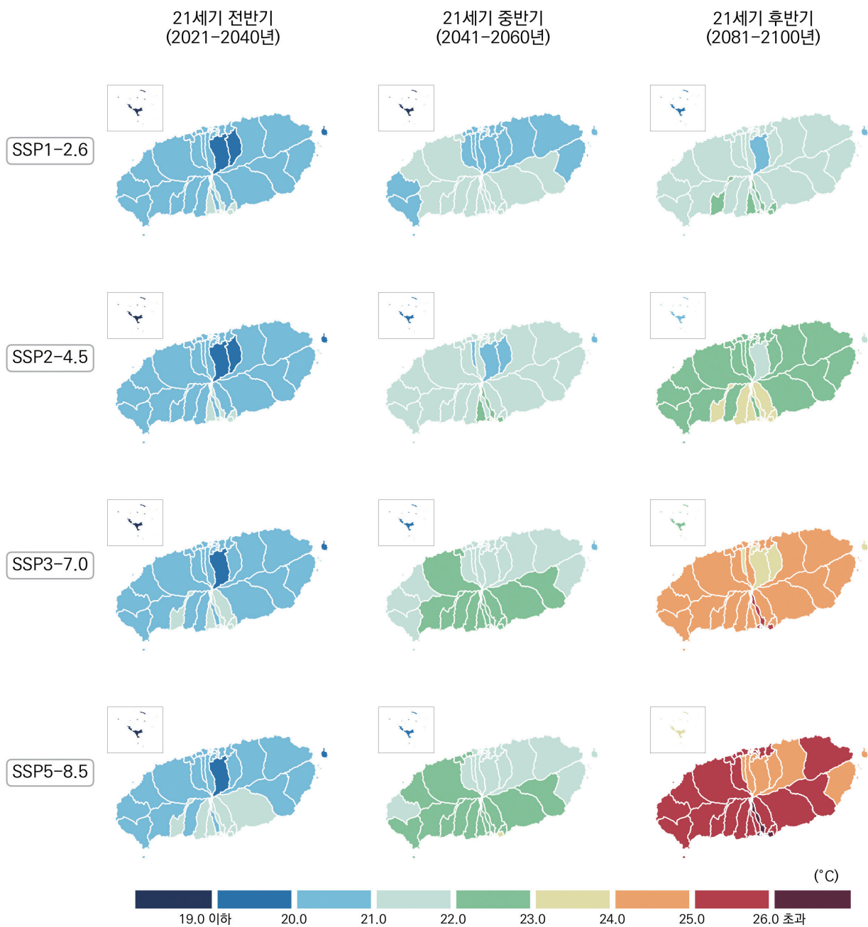
그림 4-6. 제주특별자치도의 연평균 최고기온(°C) 전망 분포도
