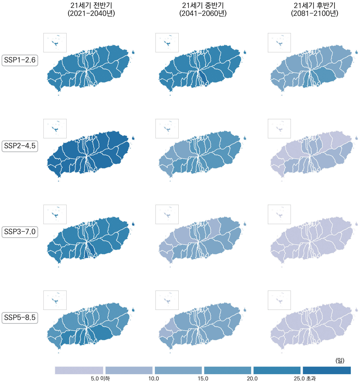
그림 4-31. 제주특별자치도의 한랭야(일) 전망 분포도
