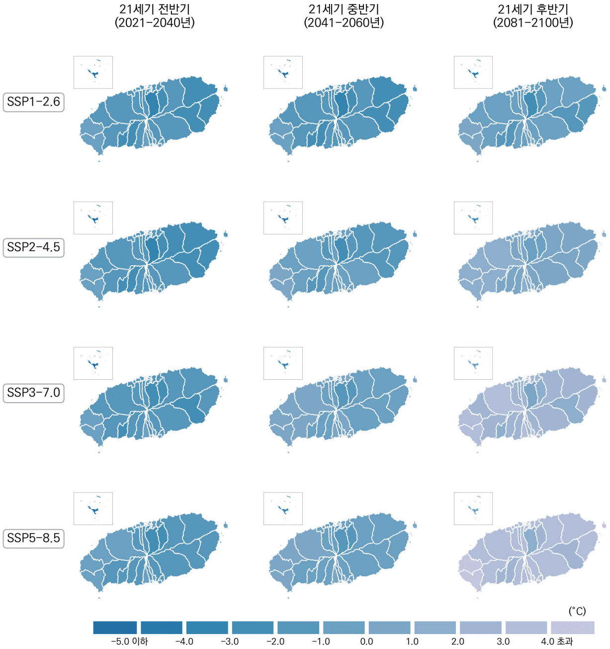
그림 4-33. 제주특별자치도의 일최저기온 연최소(°C) 전망 분포도
