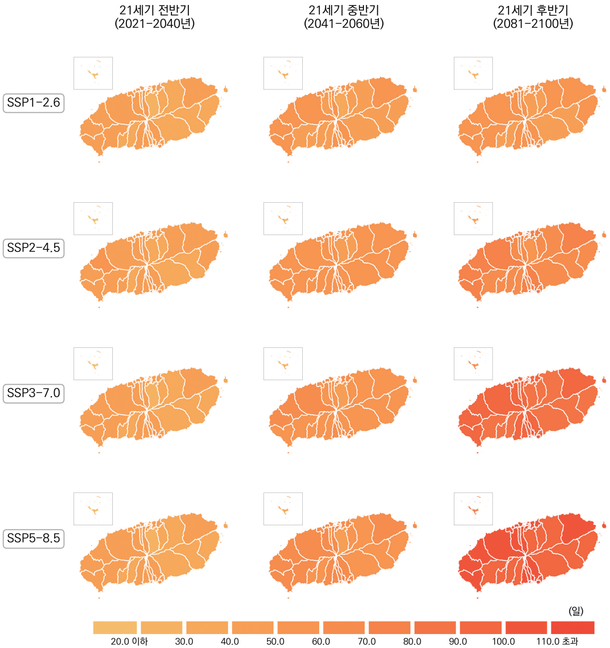
그림 4-19. 제주특별자치도의 열대야일수(일) 전망 분포도
