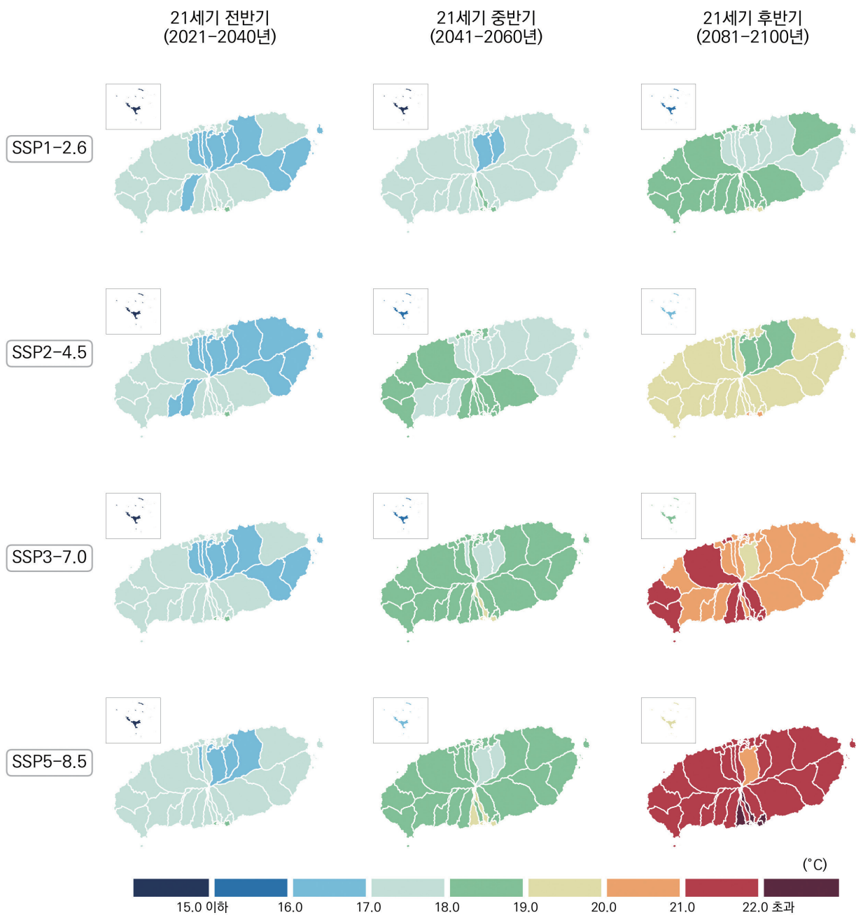
그림 4-1. 제주특별자치도의 연평균기온(°C) 전망 분포도
