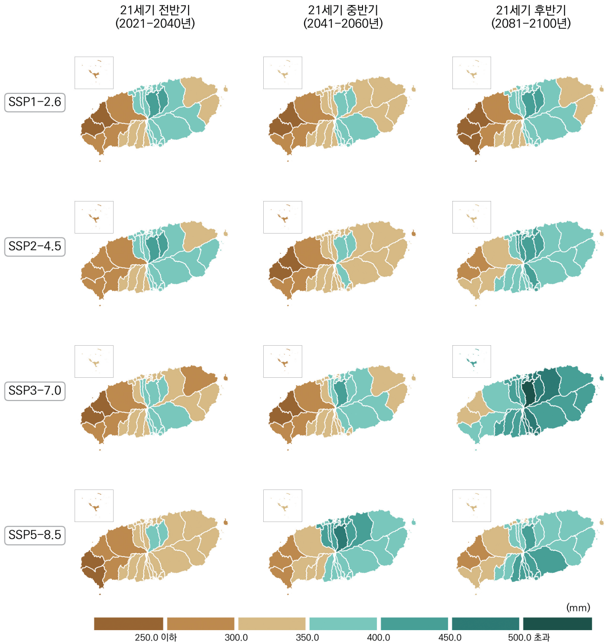
그림 4-37. 제주특별자치도의 5일최다강수량(mm) 전망 분포도
