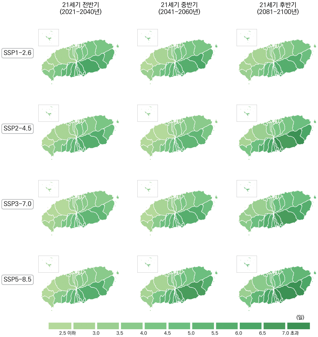
그림 4-34. 제주특별자치도의 호우일수(일) 전망 분포도
