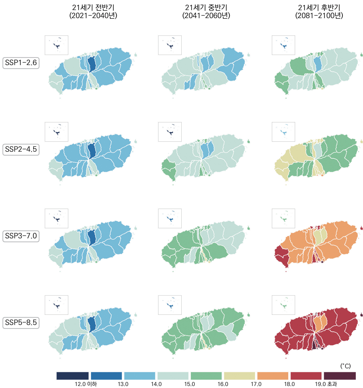
그림 4-11. 제주특별자치도의 연평균 최저기온(°C) 전망 분포도
