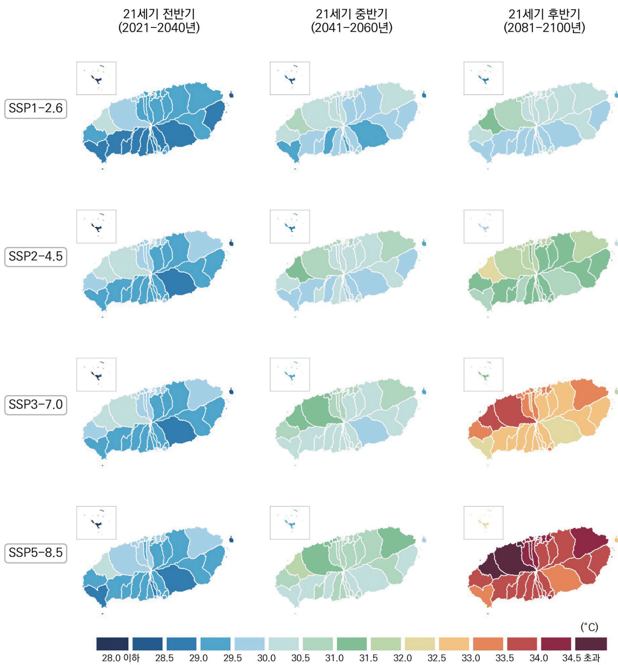
그림 4-8. 제주특별자치도의 여름철 연평균 최고기온(°C) 전망 분포도
