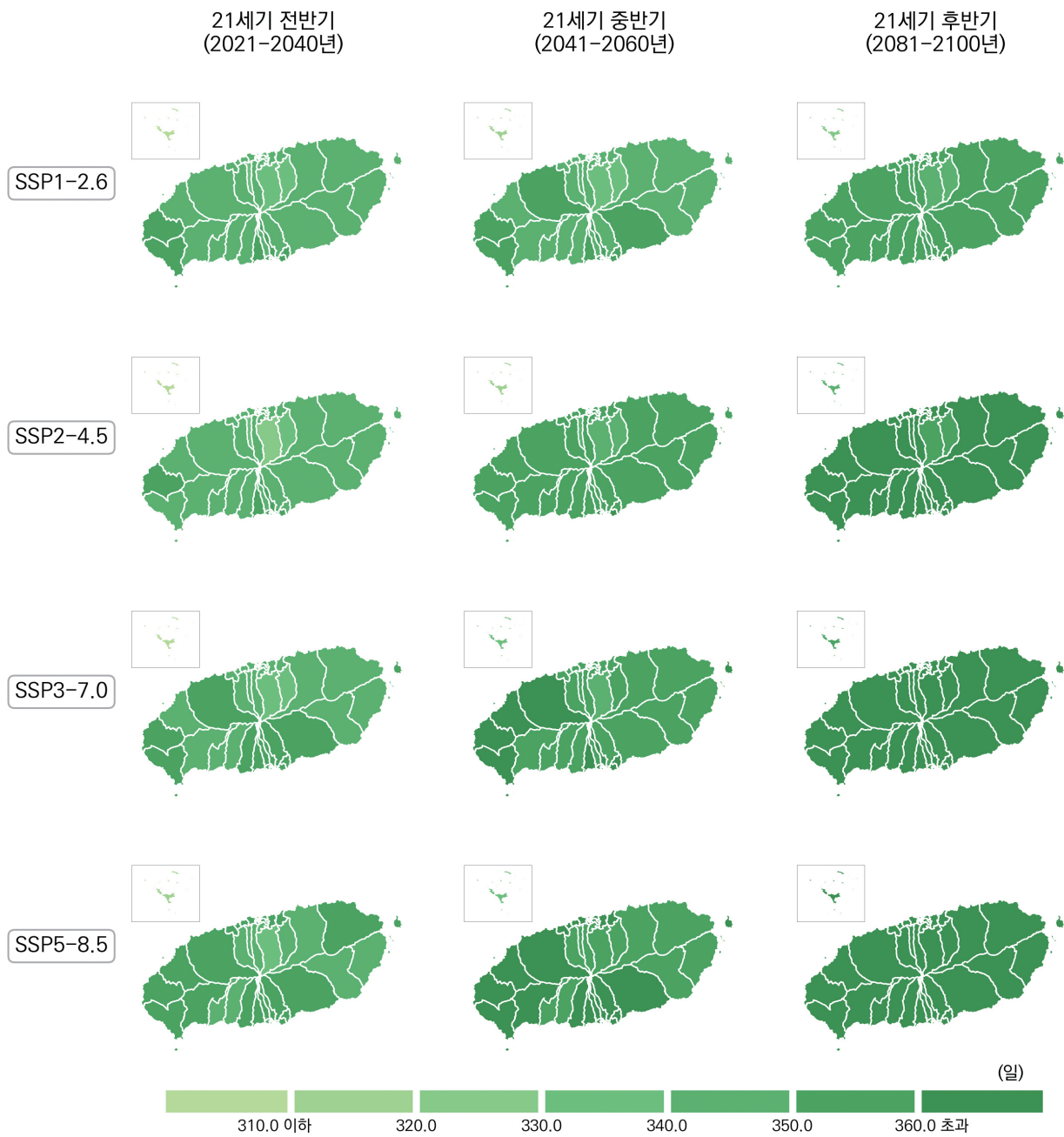
그림 4-26. 제주특별자치도의 식물성장가능기간(일) 전망 분포도
