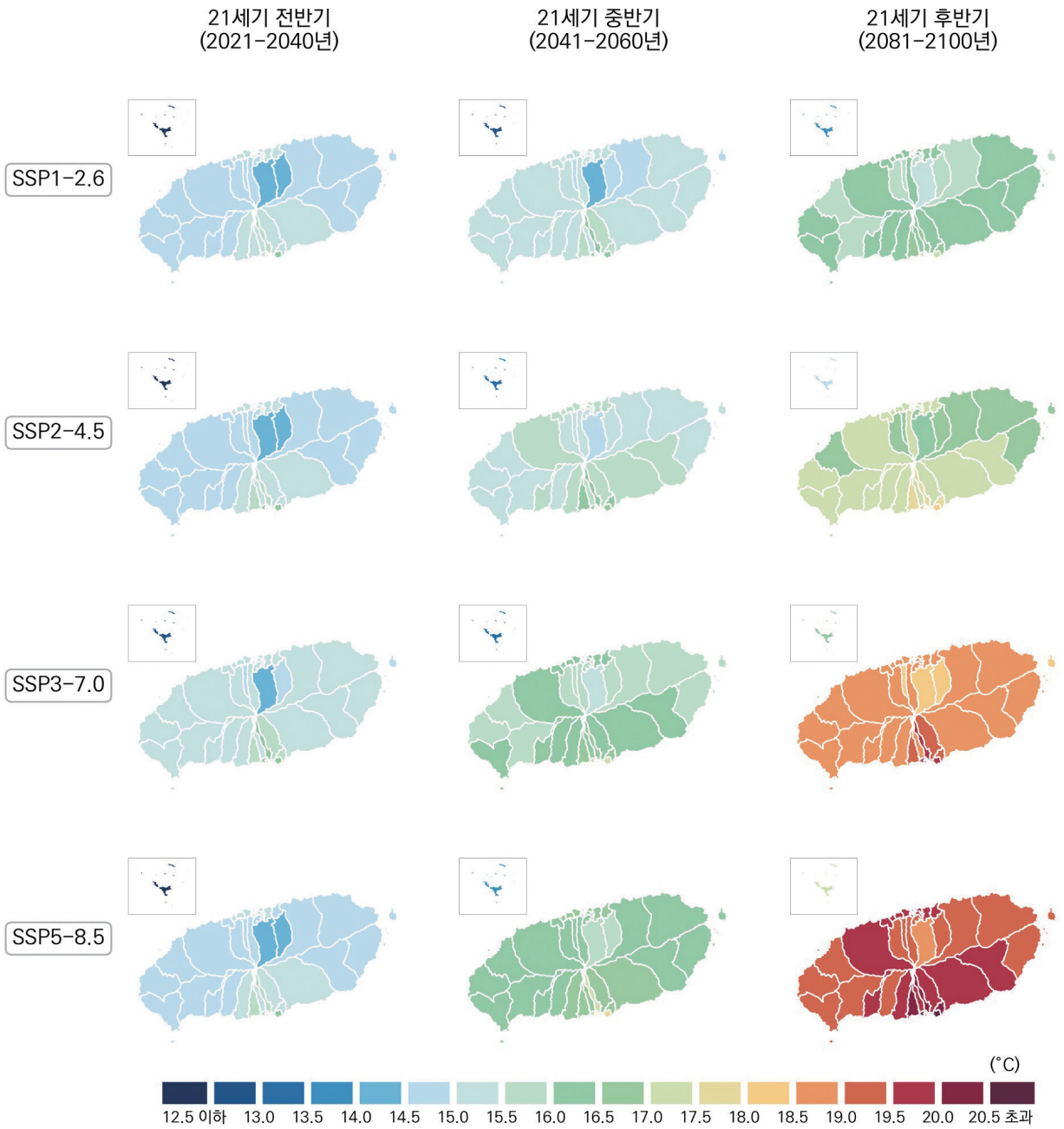
그림 4-2. 제주특별자치도의 봄철 연평균기온(°C) 전망 분포도
