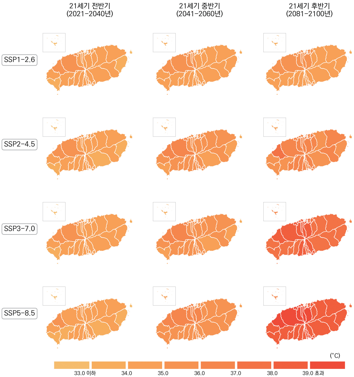
그림 4-23. 제주특별자치도의 일최고기온 연최대(°C) 전망 분포도
