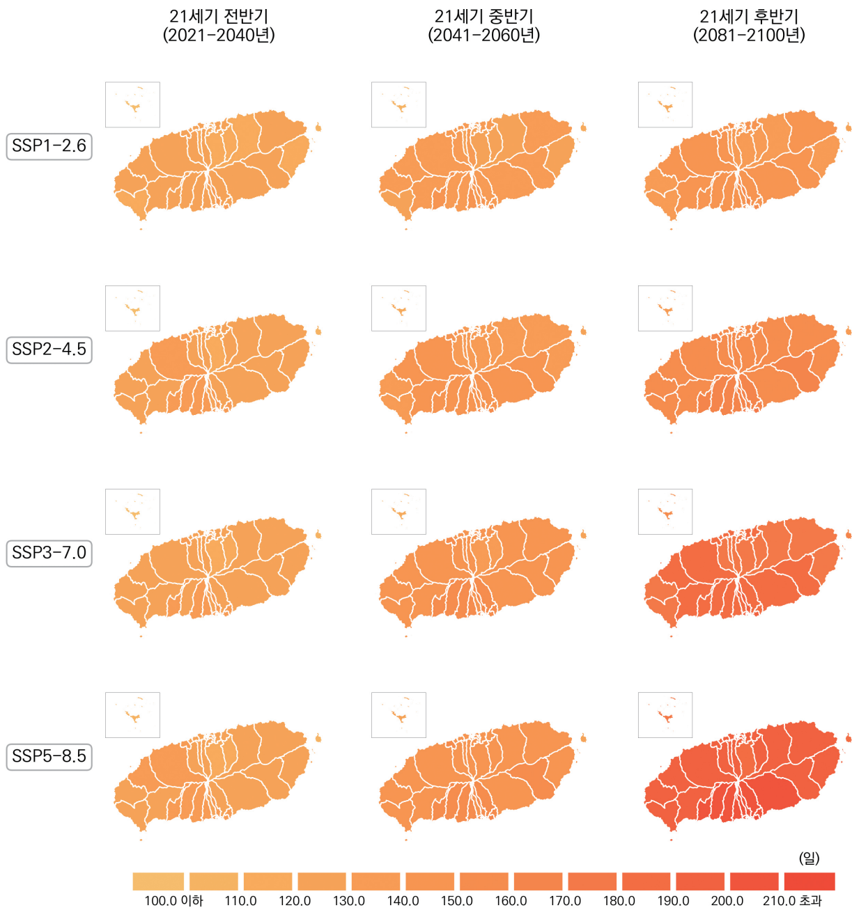
그림 4-20. 제주특별자치도의 여름일수(일) 전망 분포도
