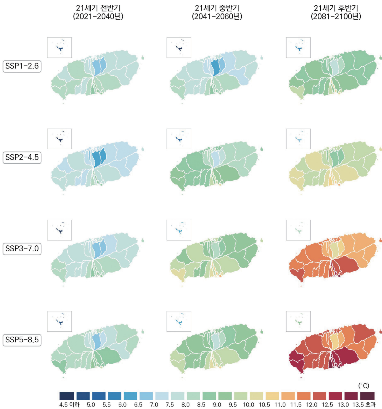
그림 4-5. 제주특별자치도의 겨울철 연평균기온(°C) 전망 분포도
