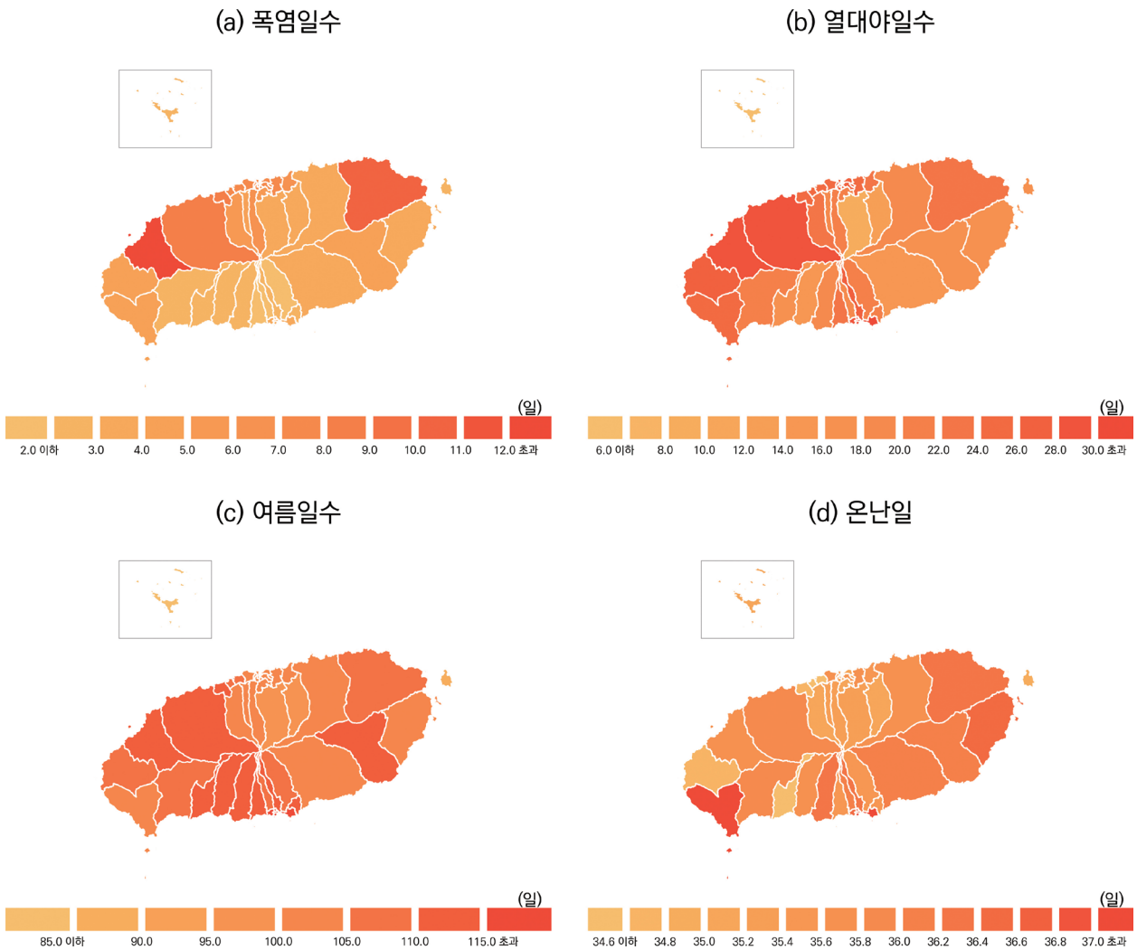
그림 3-2. 현재(2000-2019년) 제주특별자치도 고온 관련 극한기후지수 분포
