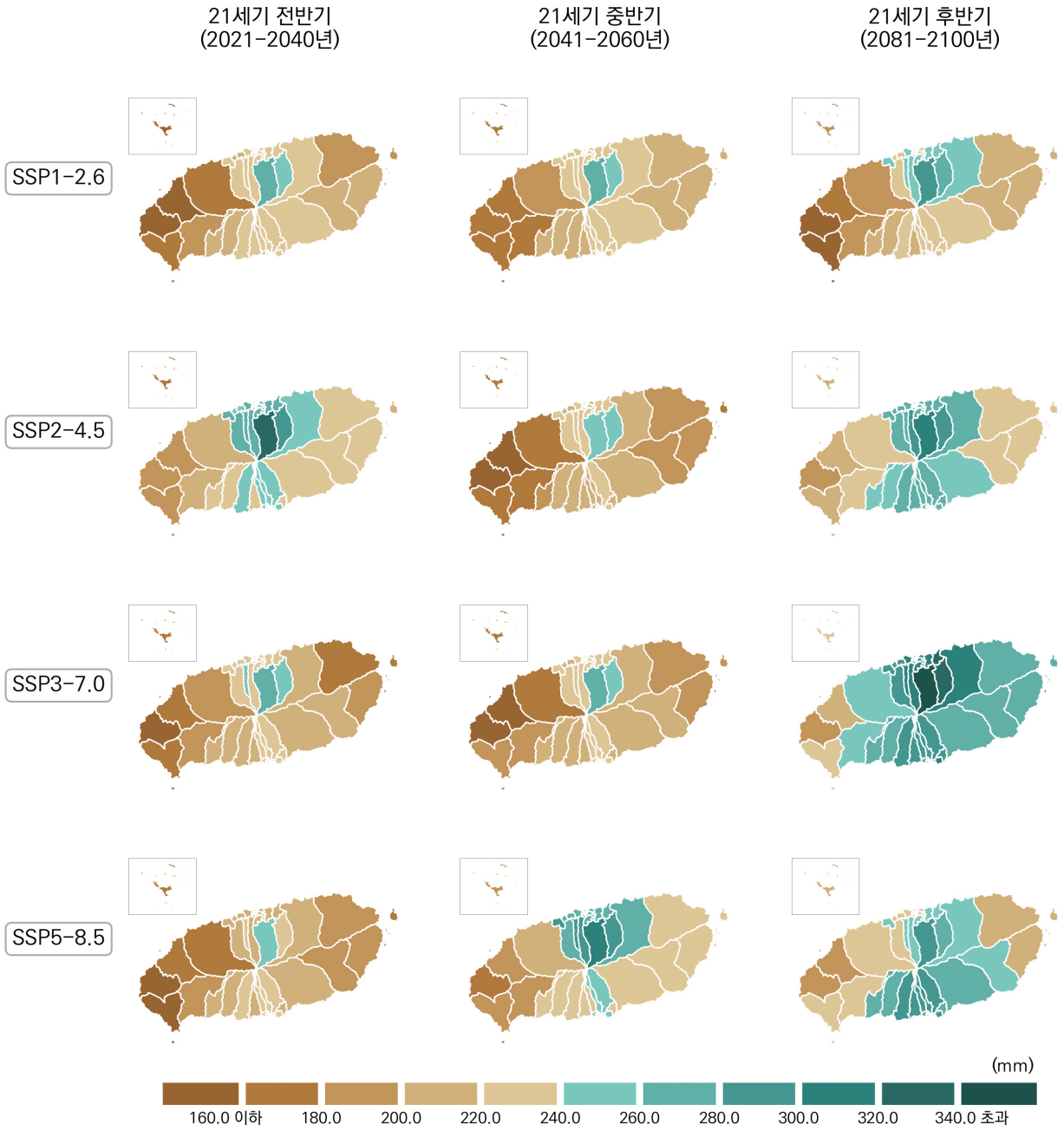
그림 4-36. 제주특별자치도의 1일최다강수량(mm) 전망 분포도
