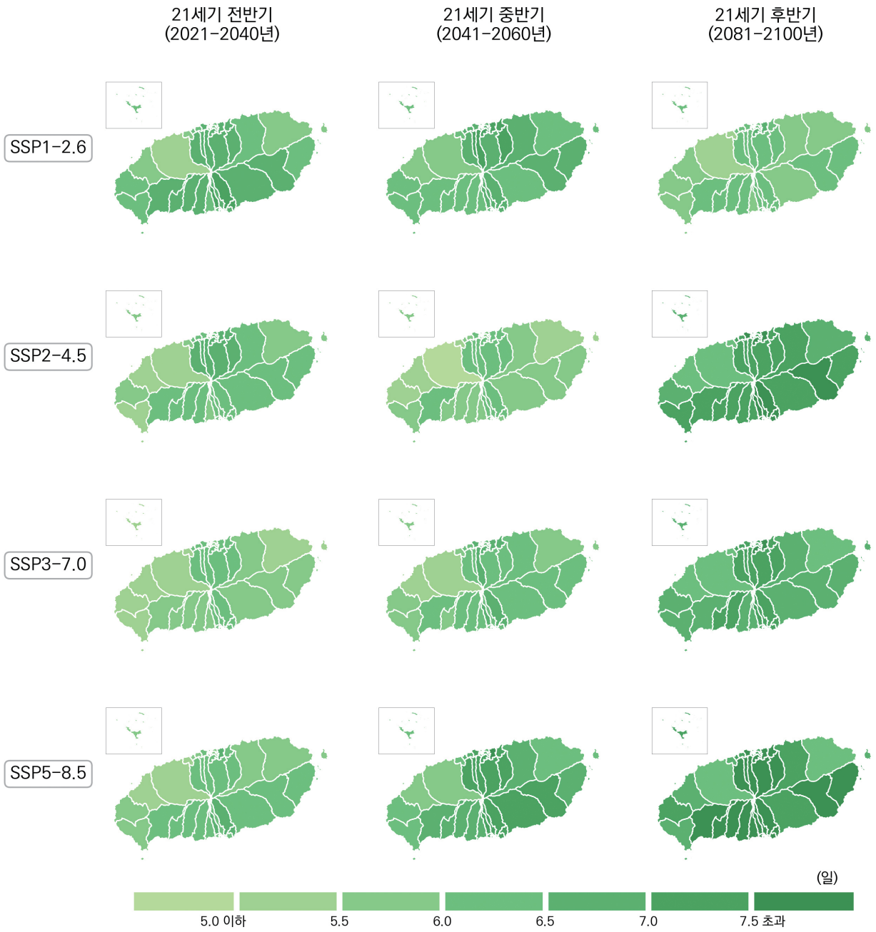
그림 4-38. 제주특별자치도의 95퍼센타일강수일수(일) 전망 분포도
