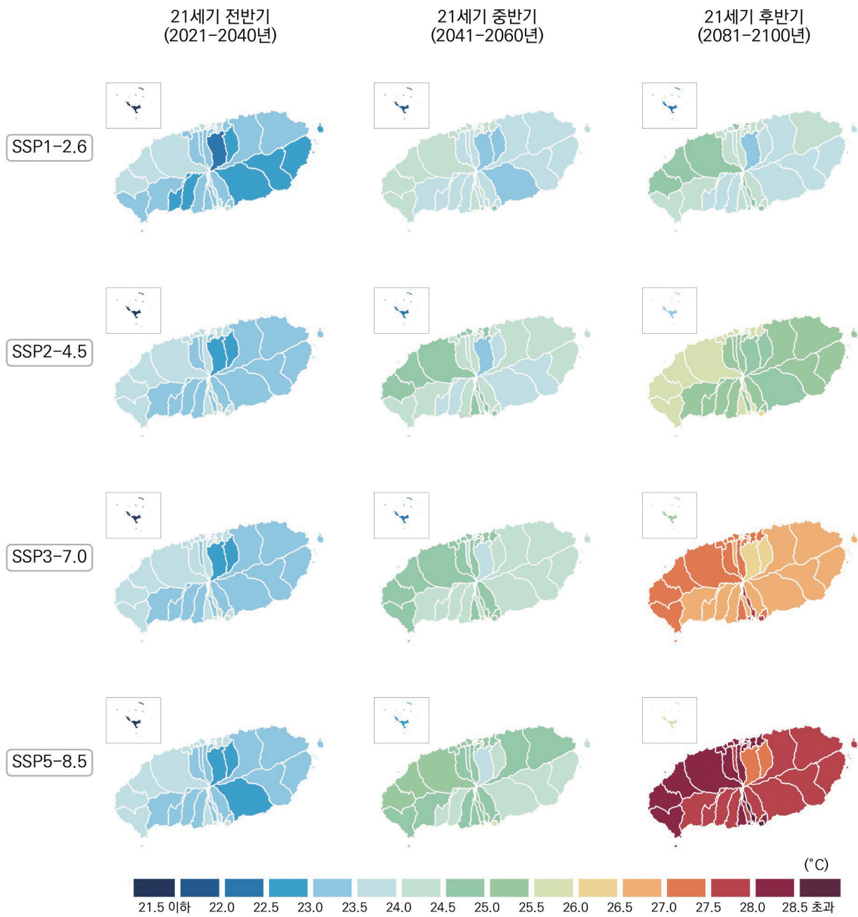
그림 4-13. 제주특별자치도의 여름철 연평균 최저기온(°C) 전망 분포도
