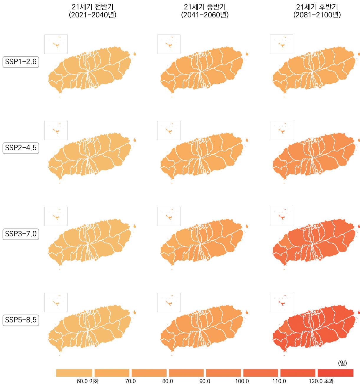
그림 4-22. 제주특별자치도의 온난야(일) 전망 분포도
